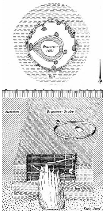
Walsum-Vierlinden: Germanischer Brunnenschacht südlich des ehemaligen Maashofes. Oben Aufsicht auf die Brunnenkonstruktion, unten Schnitt durch die Brunnengrube. Abb. 3
