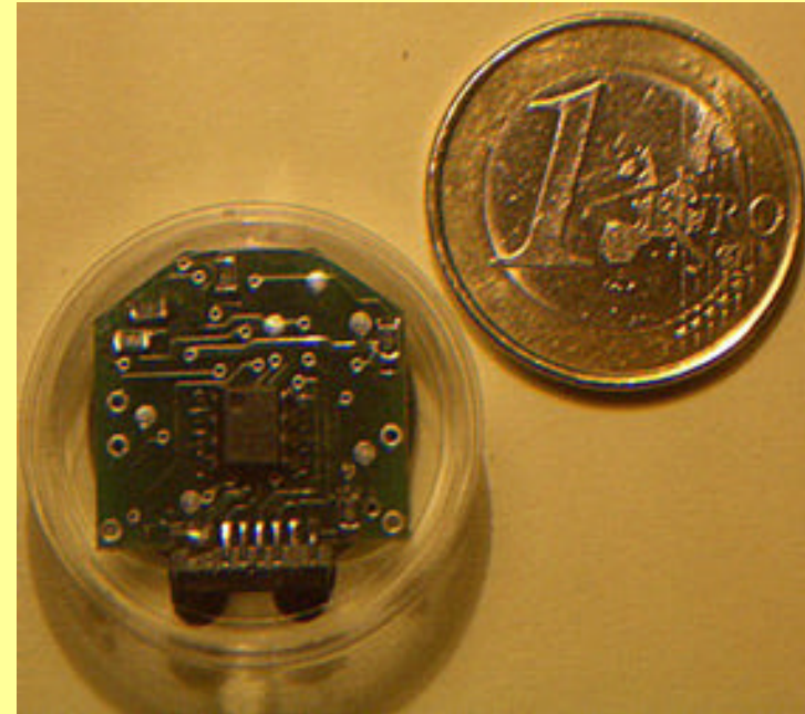
Elektronischer Temperaturschreiber (insbesondere für weiterführende Schulen)
